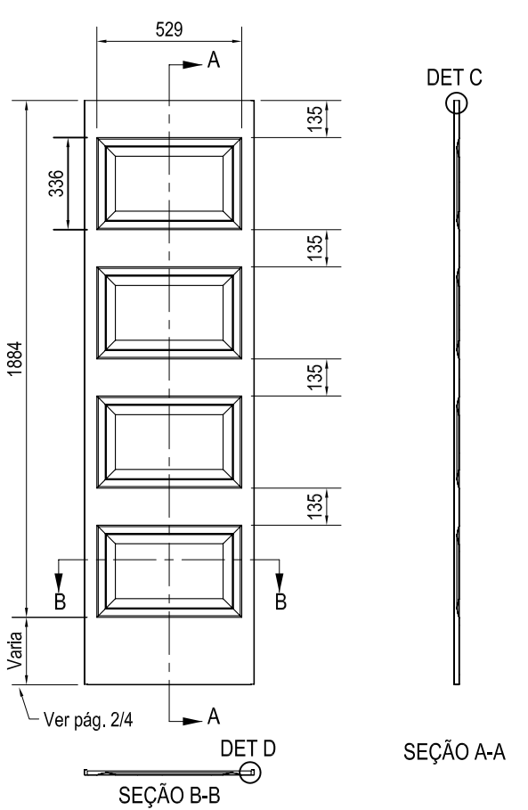
Desenho técnico do Painel de Almofoada Horizontal
