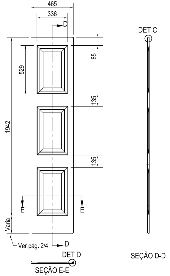
Desenho técnico do Painel de Almofoada Vertical
